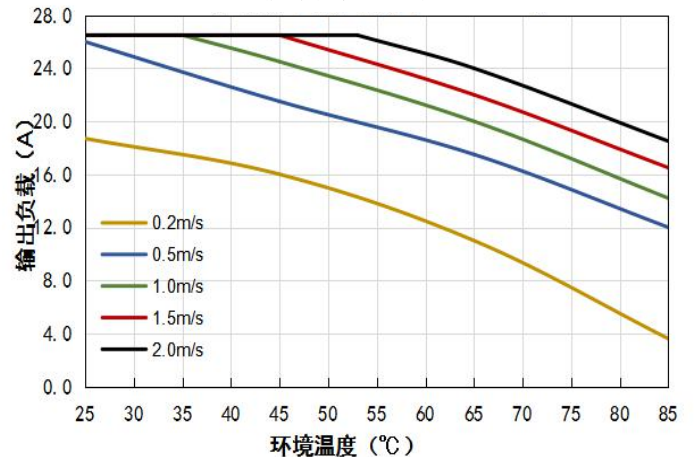
VCF4815QBO-400WFR3(-N) 温度降额曲线 (Vin=48V)
