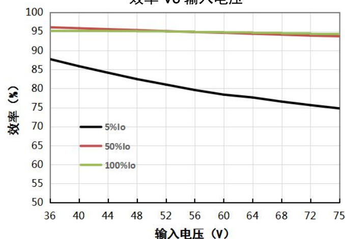
VCF4828QBO-400W(F/H)R3(-N) 效率 VS 输入电压
