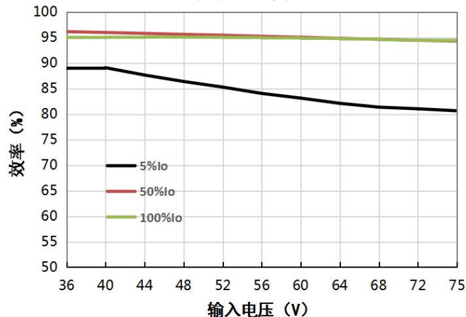
VCF4824QBO-400W(F/H)R3(-N) 效率 VS 输入电压
