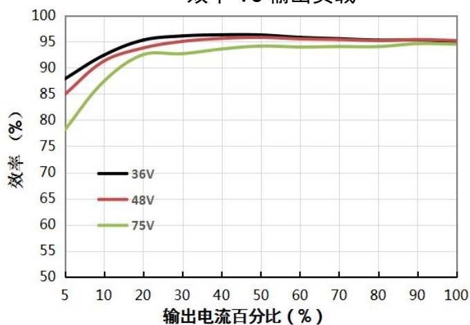
VCF4815QBO-400W(F/H)R3(-N) 效率 VS 输出负载
