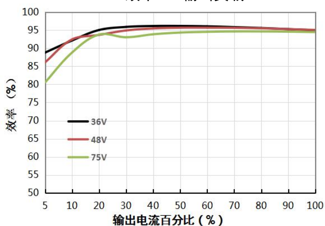
VCF4824QBO-400W(F/H)R3(-N) 效率 VS 输出负载
