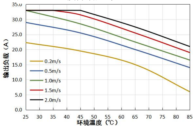
VCF4812QBO-400WFR3(-N) 温度降额曲线 (Vin=48V)
