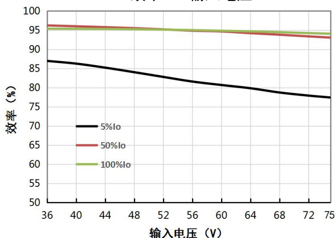
VCF4815QBO-400W(F/H)R3(-N) 效率 VS 输入电压
