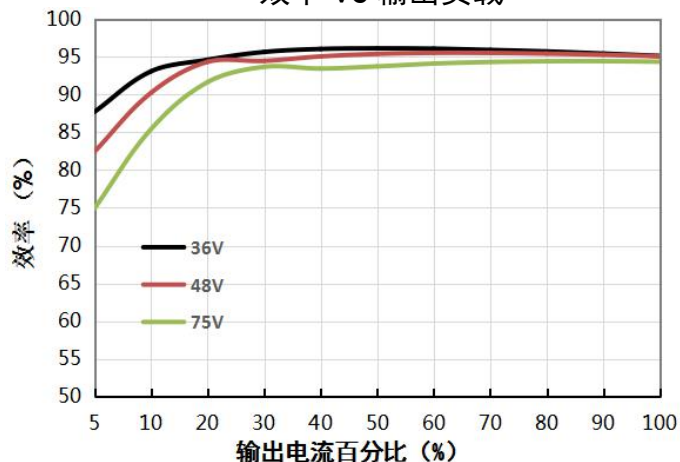
VCF4828QBO-400W(F/H)R3(-N) 效率 VS 输出负载
